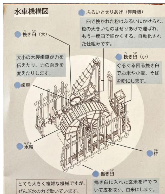
水車機構図
